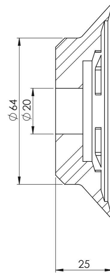
SEZIONE B-B
